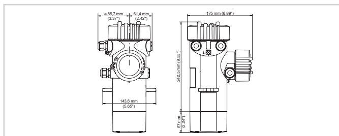
Размеры MINITRAC 31
