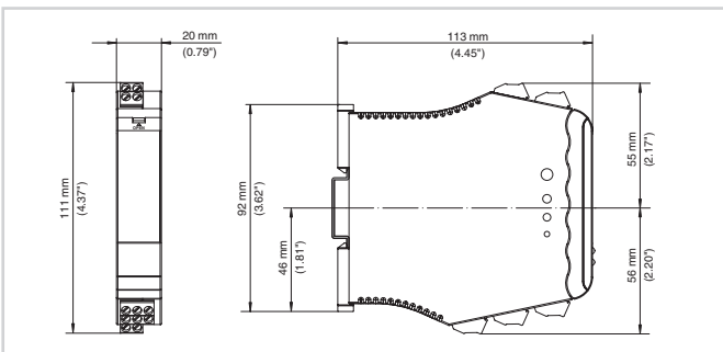
Размеры VEGATOR 122
